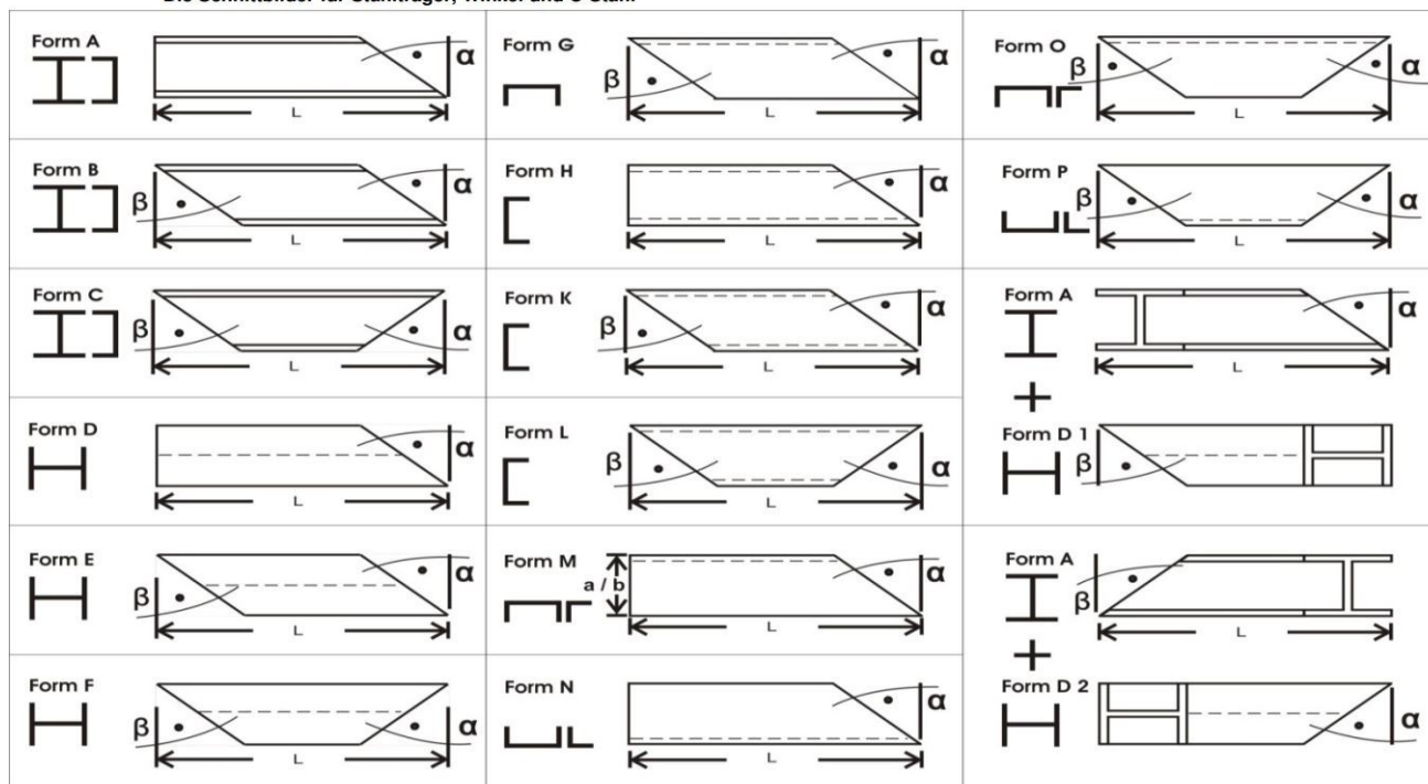
Die Schnittbilder für Stahlträger, Winkel und U-Stahl
